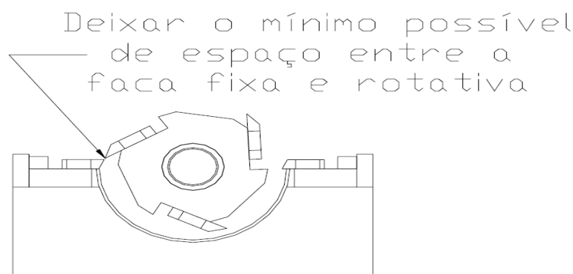
Figura 4 – Espaçamento entre Facas
