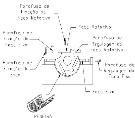
Figura 6 – Peças de reposição:
